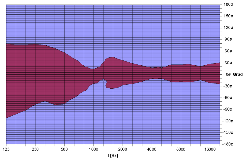
TSM 15 Vertikal / - 6 dB Isobaren
