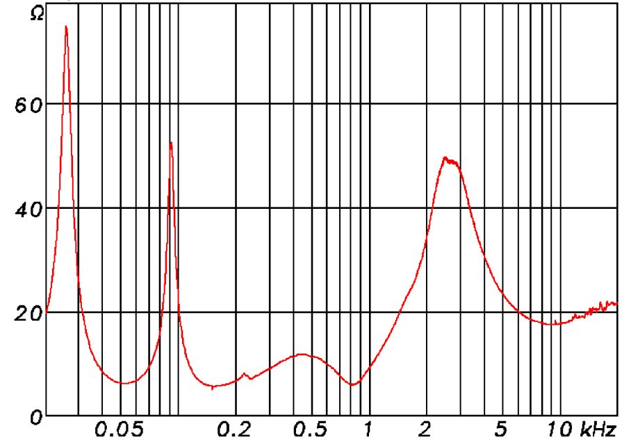
Impedance TSM15 Norm.= 8 Ohm ; Min.= 5,7 Ohm
