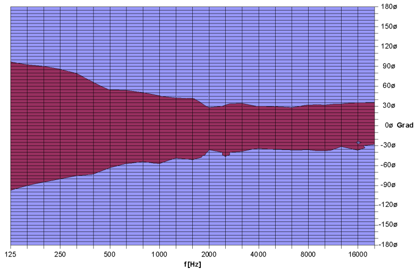
TSM 15 Horizontal / - 6 dB Isobaren
