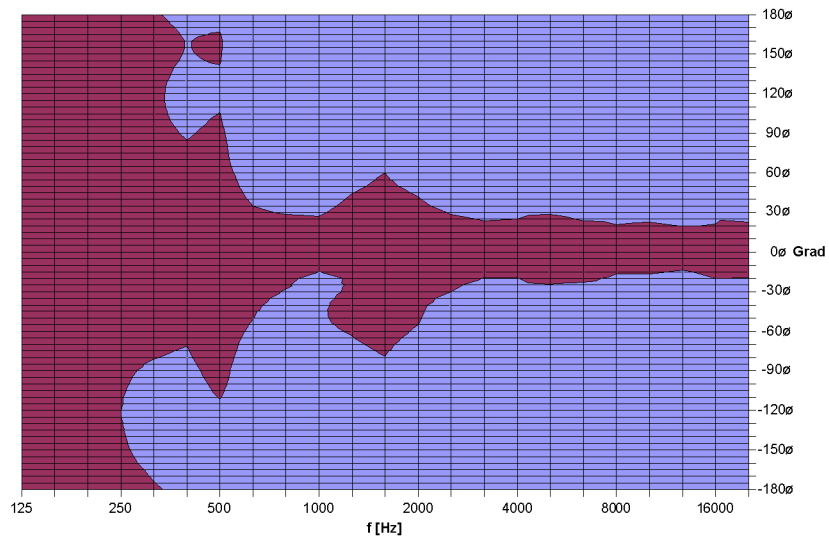
TSM12 90° x 60° Vertikal - -6 dB Isobaren
