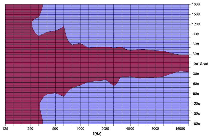
TSM 10 Horizontal / - 6 dB Isobaren
