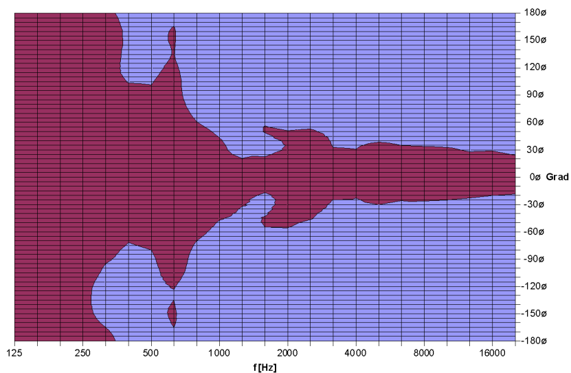
TSM 10 Vertikal / - 6 dB Isobaren
