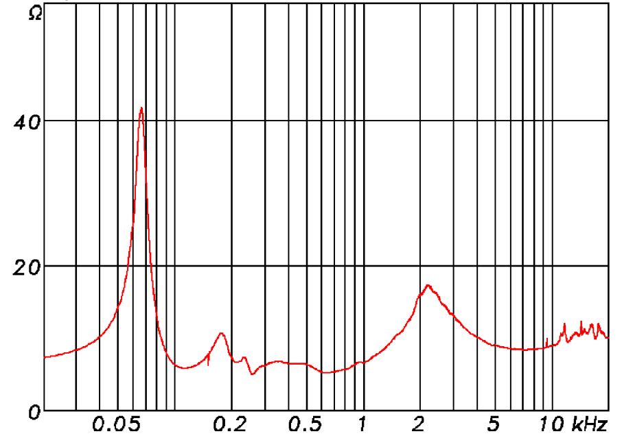
Impedance TSE4030 Norm.= 8 Ohm ; Min.= 5, 0 Ohm
