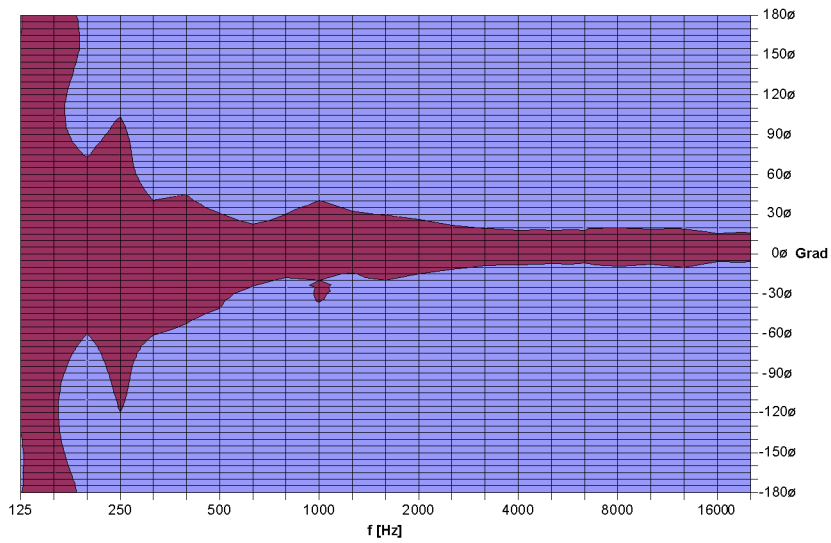
TSE 4030 Vertikal / - 6 dB Isobaren
