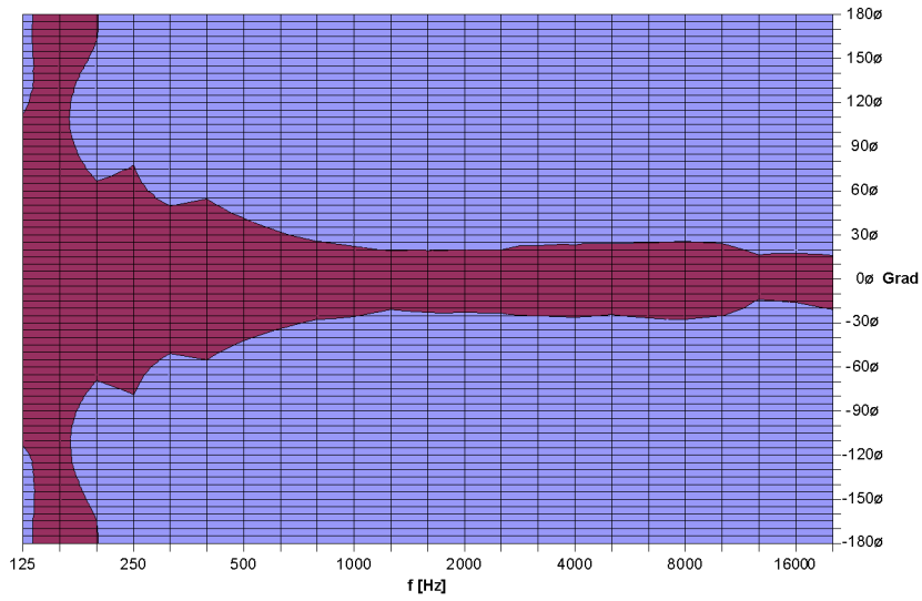
TSE 4030 Horizontal / - 6 dB Isobaren
