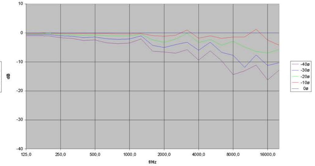
M5 Horizontal - Frequenzgang Off Axis-
