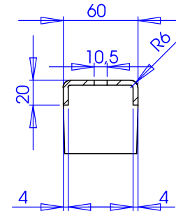
SCHNITT A-A MAßSTAB 1 : 3
