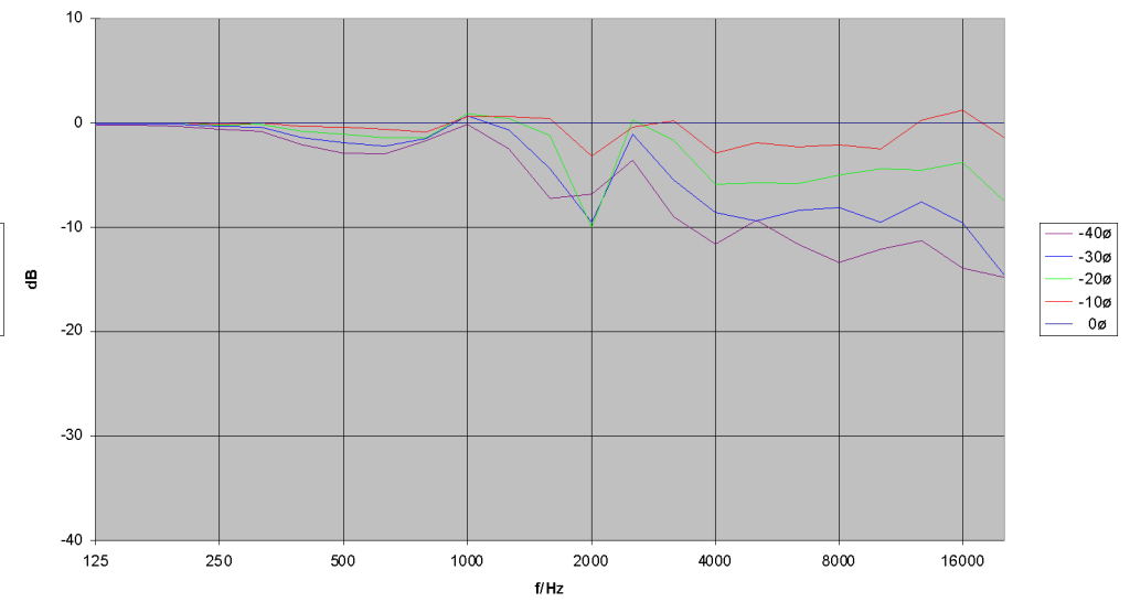
TSMini Vertikal - Frequenzgang Off Axis (-)
