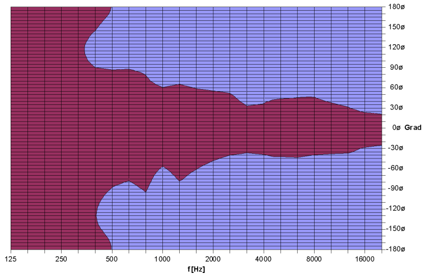
TSMini Horizontal / - 6 dB Isobaren
