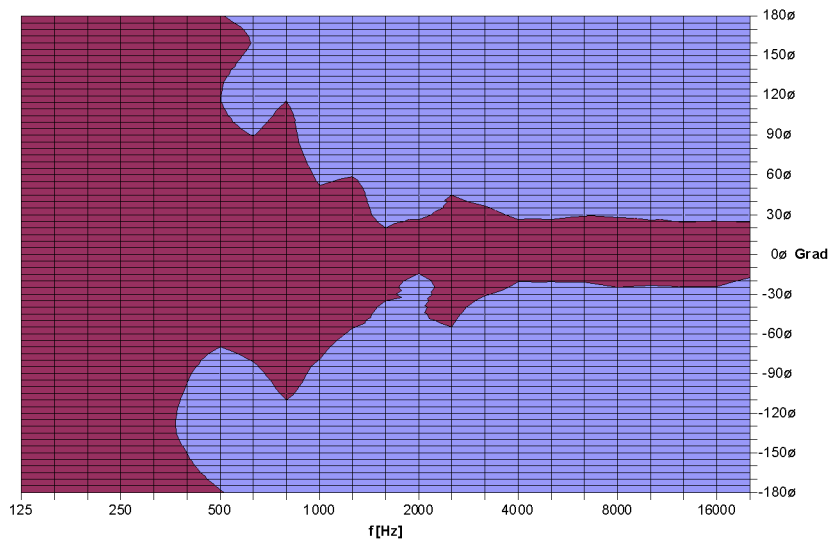
TSMini Vertikal / - 6 dB Isobaren
