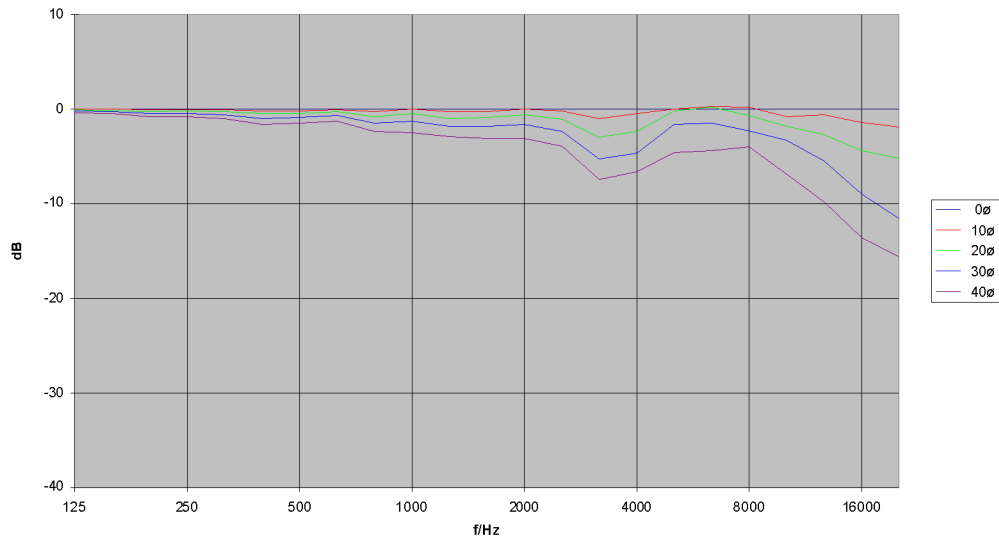
TSMini Horizontal - Frequenzgang Off Axis (+)
