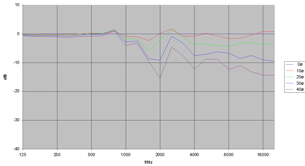
TSMini Vertikal - Frequenzgang Off Axis (+)
