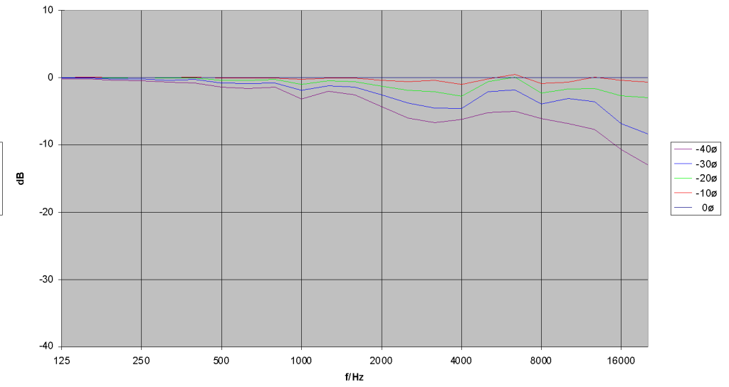
TSMini Horizontal - Frequenzgang Off Axis (-)
