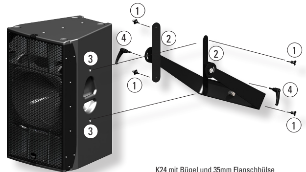
K24 mit Bügel und 35mm Flanschhülse in Groundstack Position
