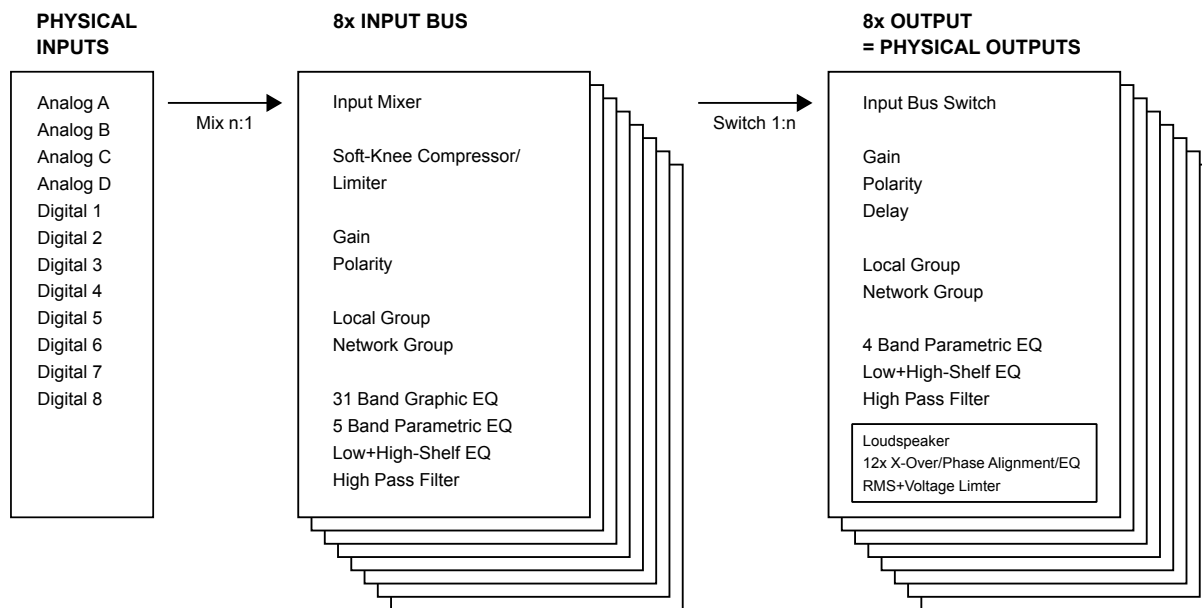
Abbildung 1.1.: Signalstruktur
